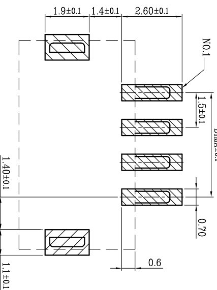
适用线路板
