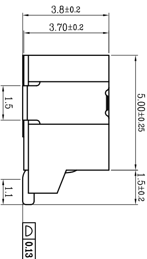
适用线路板
